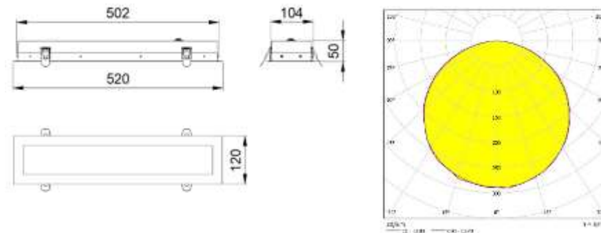
Рис.№1 Размеры светильника
