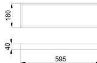
Рис.№1 Размеры светильника
