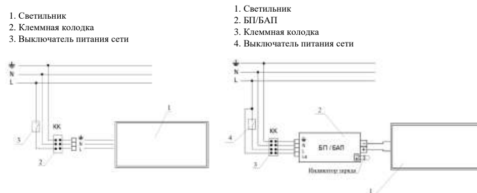
Рис. №3 Схема подключения светильника.
